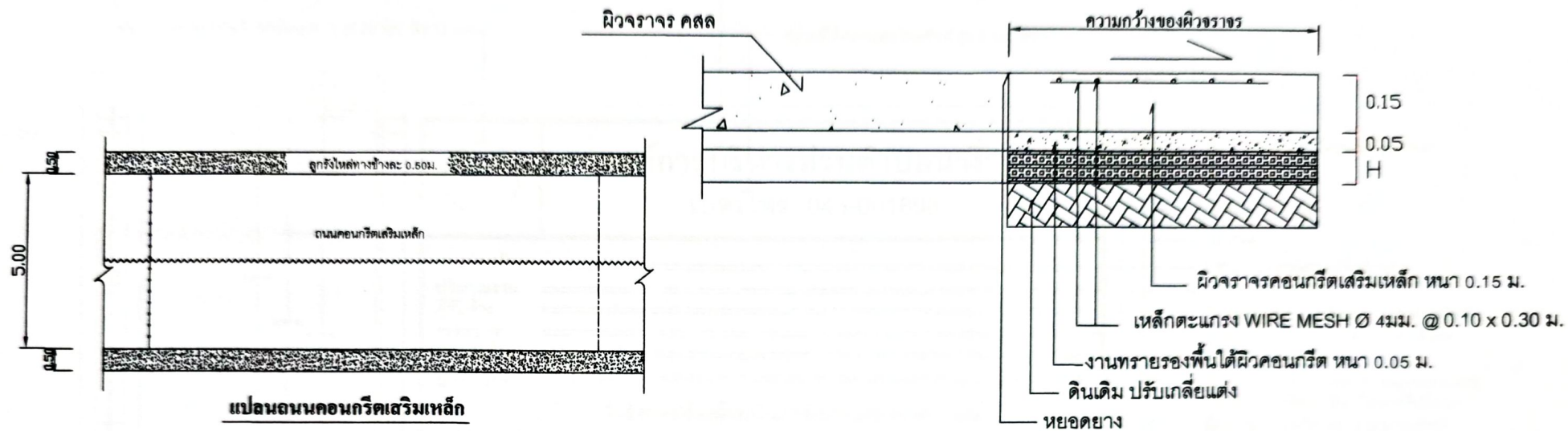
รูปตัดแสดงโครงสร้างถนนคอนกรีตเสริมเหล็ก
