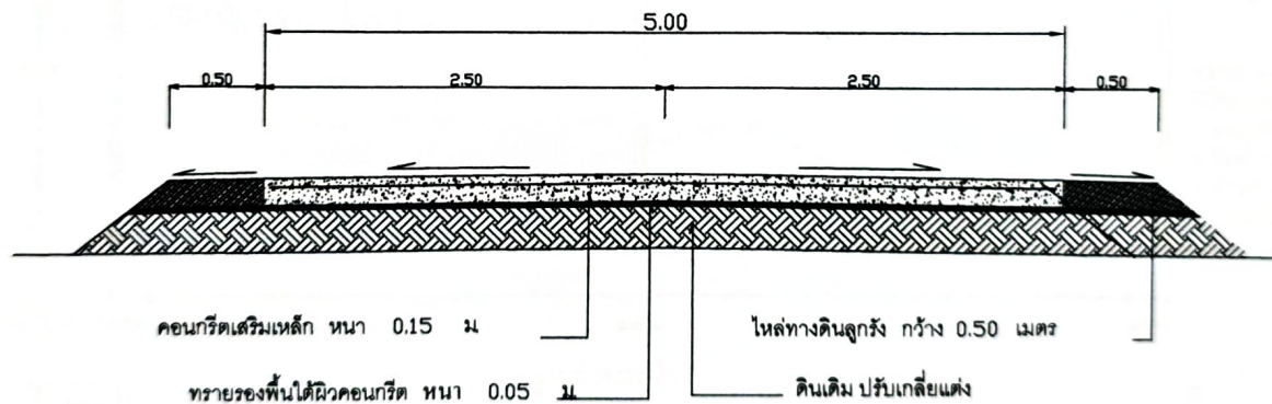
รูปตัด
